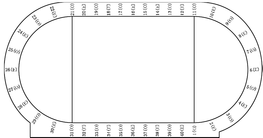
图 3 环形跑道面层厚度检验点位示意图
