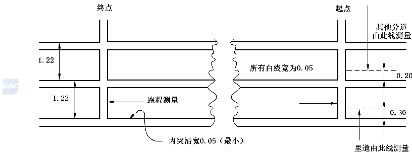
图 4 跑道长度测量点位示意图
