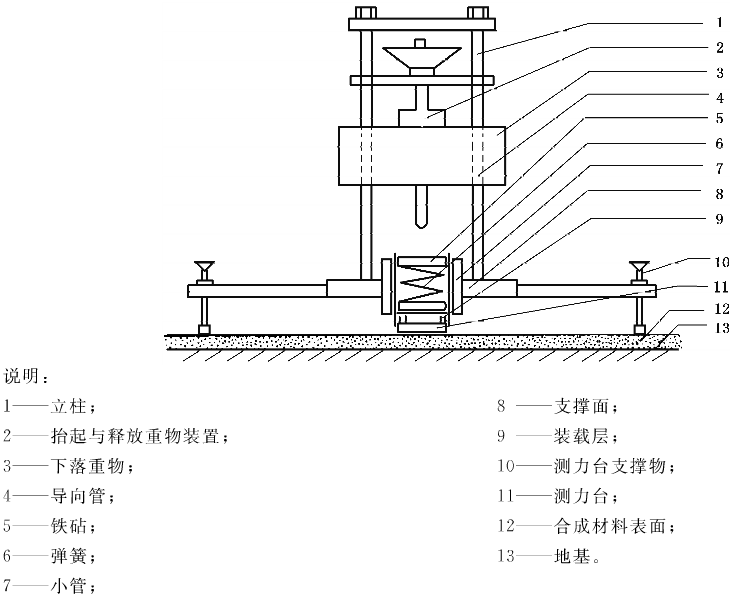
图 C.1 冲击吸收测试仪
