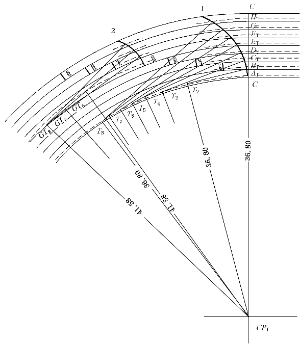
说明： 1——1 000 m、3 000 m 和 5 000 m 的起点线； 2——1 000 m、3 000 m 和 5 000 m 的分组起跑线。 注：CP 1 C——36.50 m；CP 1 A T ——36.80 m；CP 1 B T ——36.80 m + 1.12 m；CP 1 C T ……H T ——37.92 m + 每道 1.22 m；T 2 T 8 ——切线点；GT 6 GT 8 ——分组起跑线的切线点。
