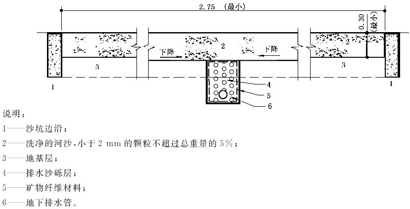
图 A.13 跳远和三级跳远设施落地区
