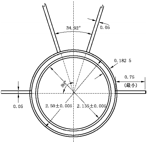
图 A.20 掷链球与掷铁饼共用投掷圈
