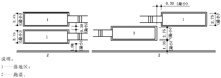
图 A.14 两个平行的跳远与三级跳远设施间的最小距离
