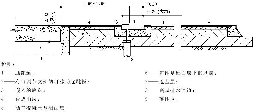
图 A.12 跳远和三级跳远设施用于起跳板嵌入的底盘
