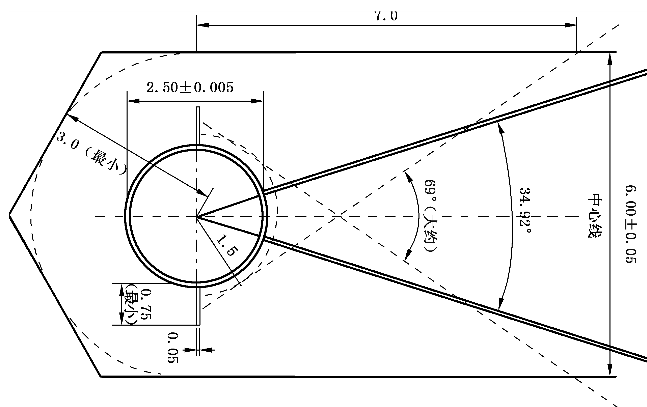
图 A.18 掷铁饼护笼
