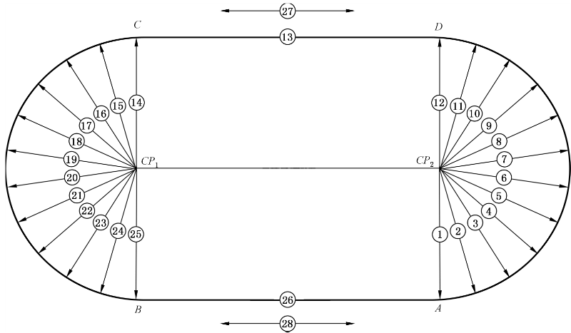
图 5 400 m 跑道精确测量点位示意图
