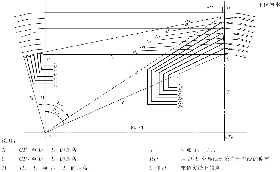
图 A.1 400 m 标准跑道 800 m 跑抢道标志线
